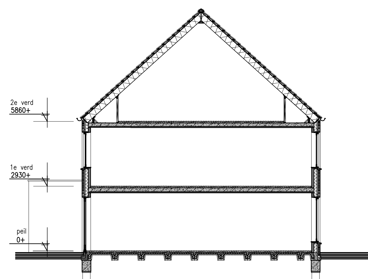
DOORSNEDE 1:100
