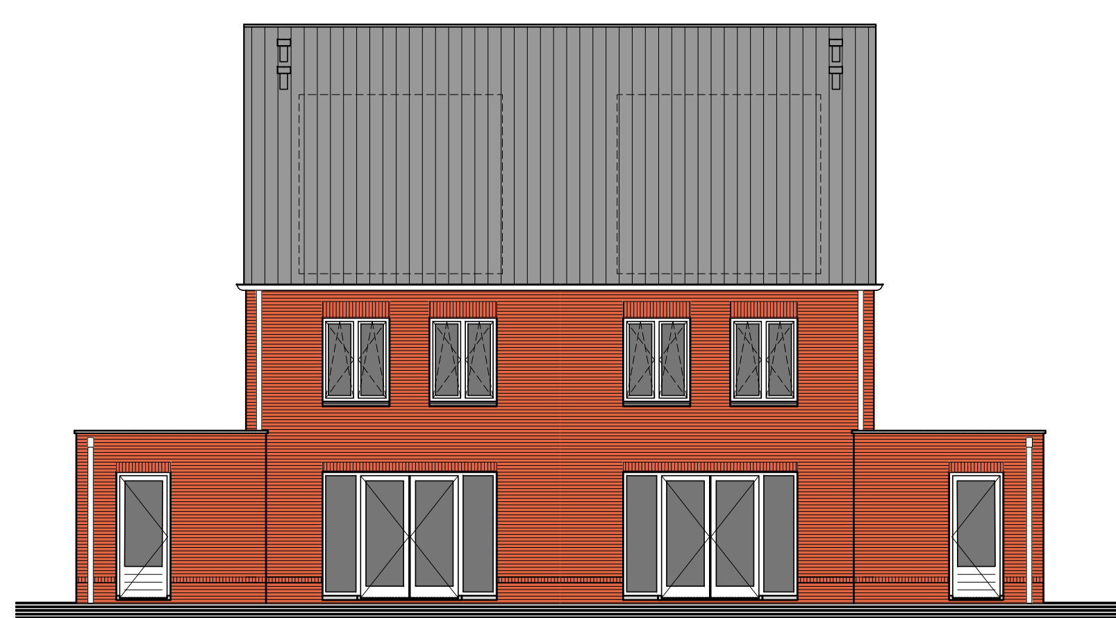
bouwnummer 12/14 Type E bouwnummer 11/13 Type E ACHTERGEVEL 1:100
