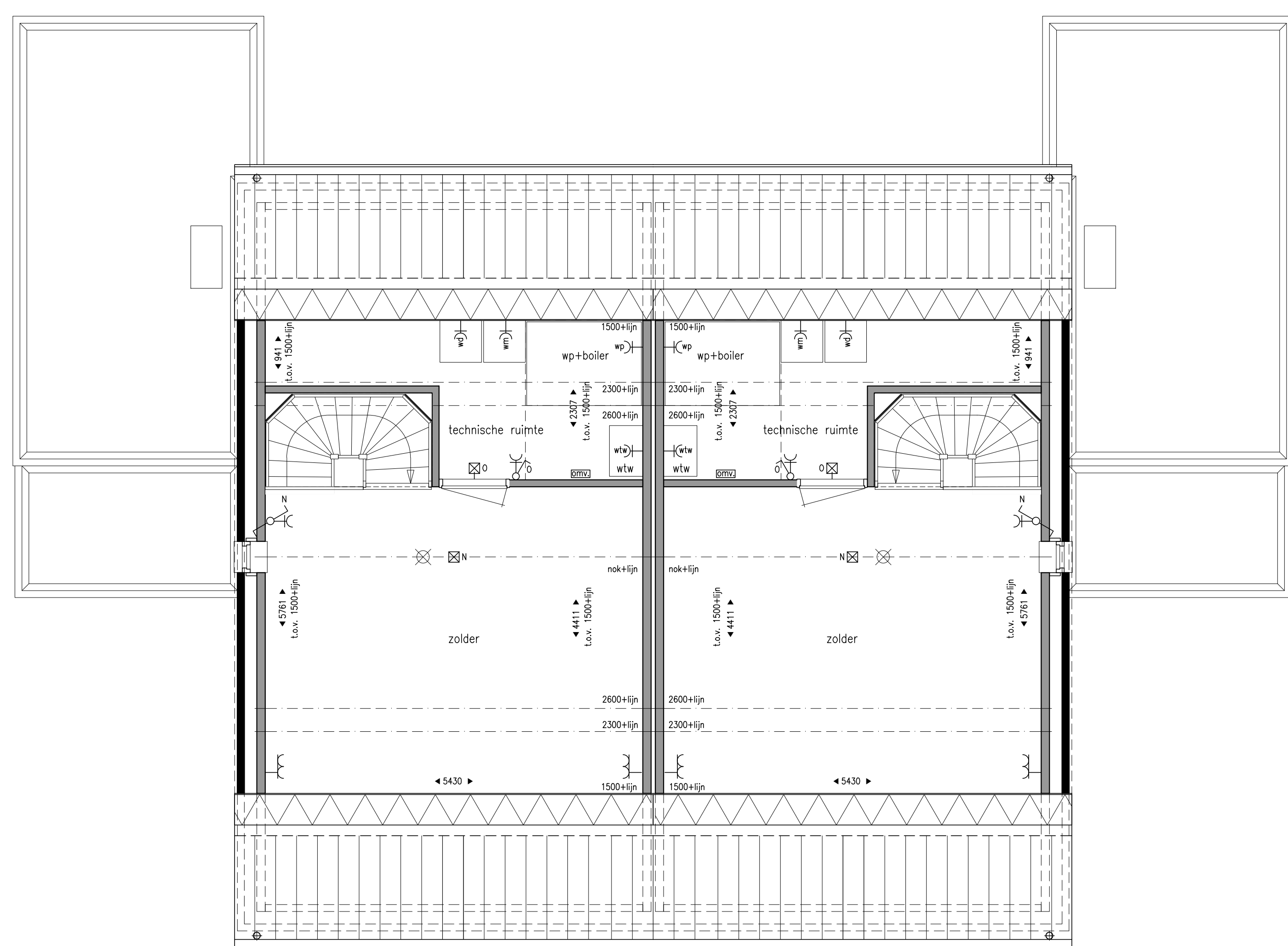
Type E Type E 2e VERDIEPING 1:50
