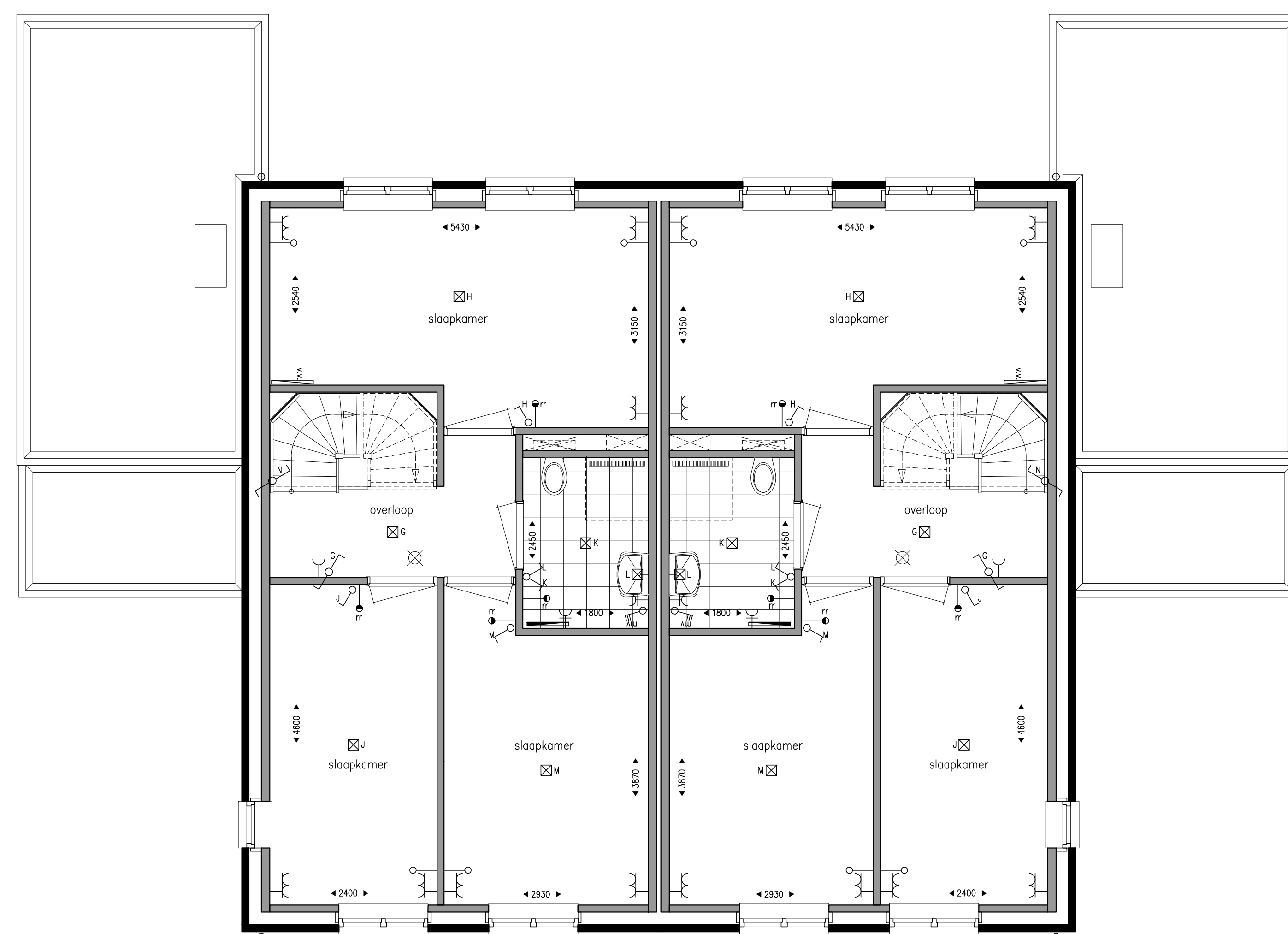
Type E Type E 1e VERDIEPING 1:50
