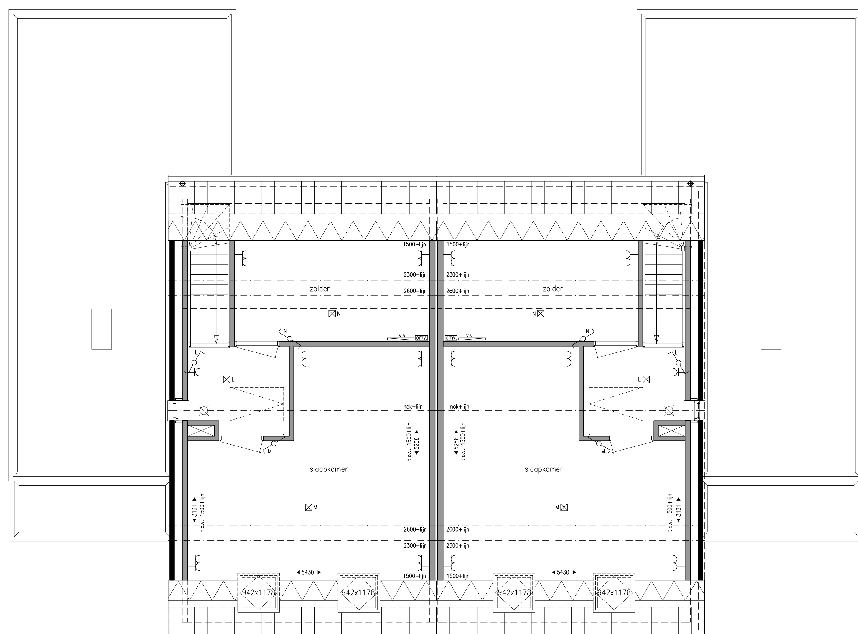
1e VERDIEPING 1:50
