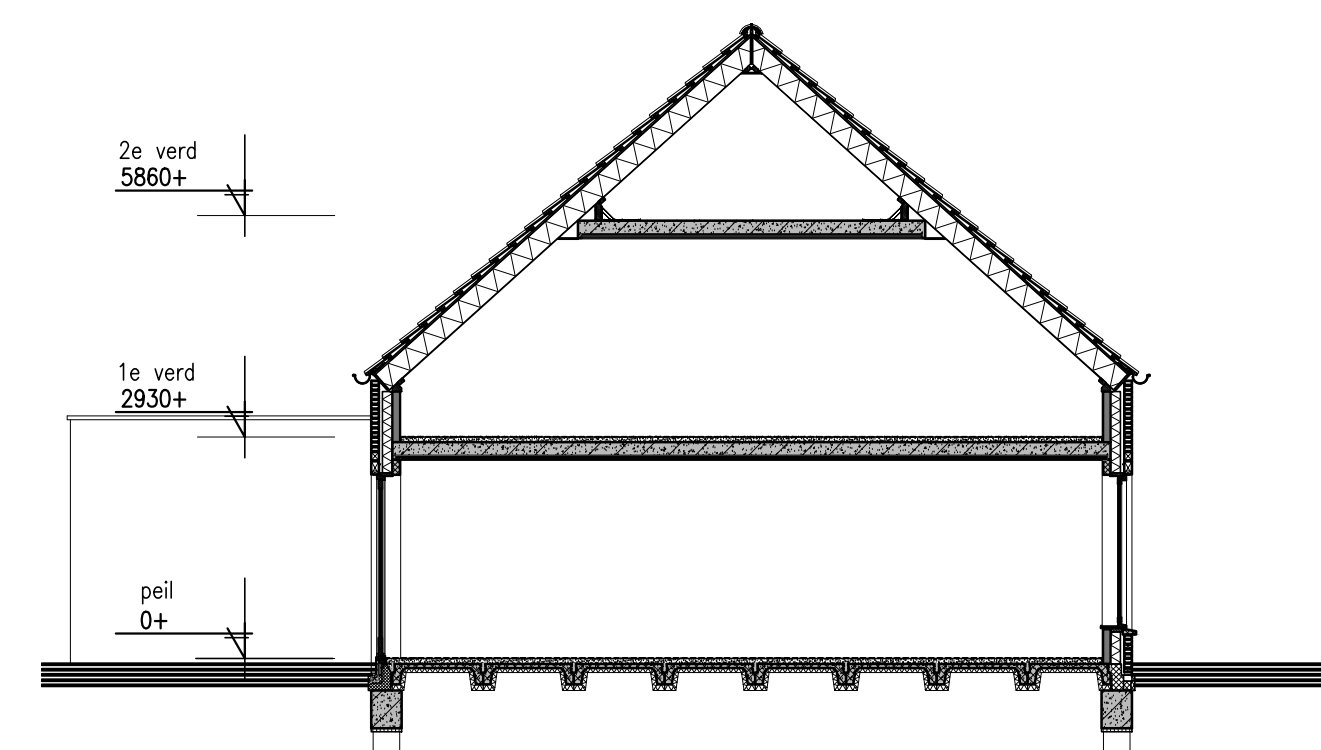
DOORSNEDE 1:100
