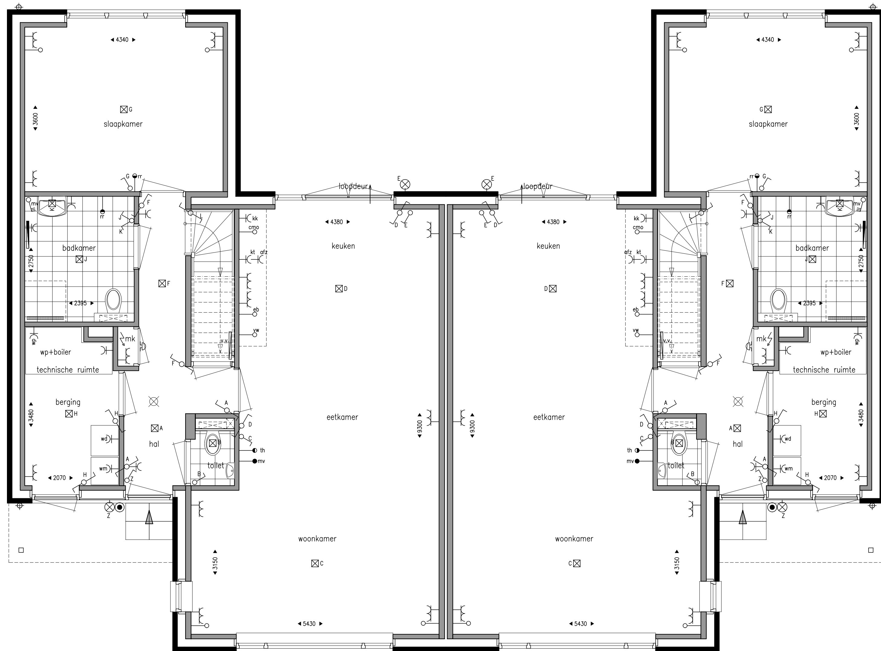
BEGANE GROND 1:50
