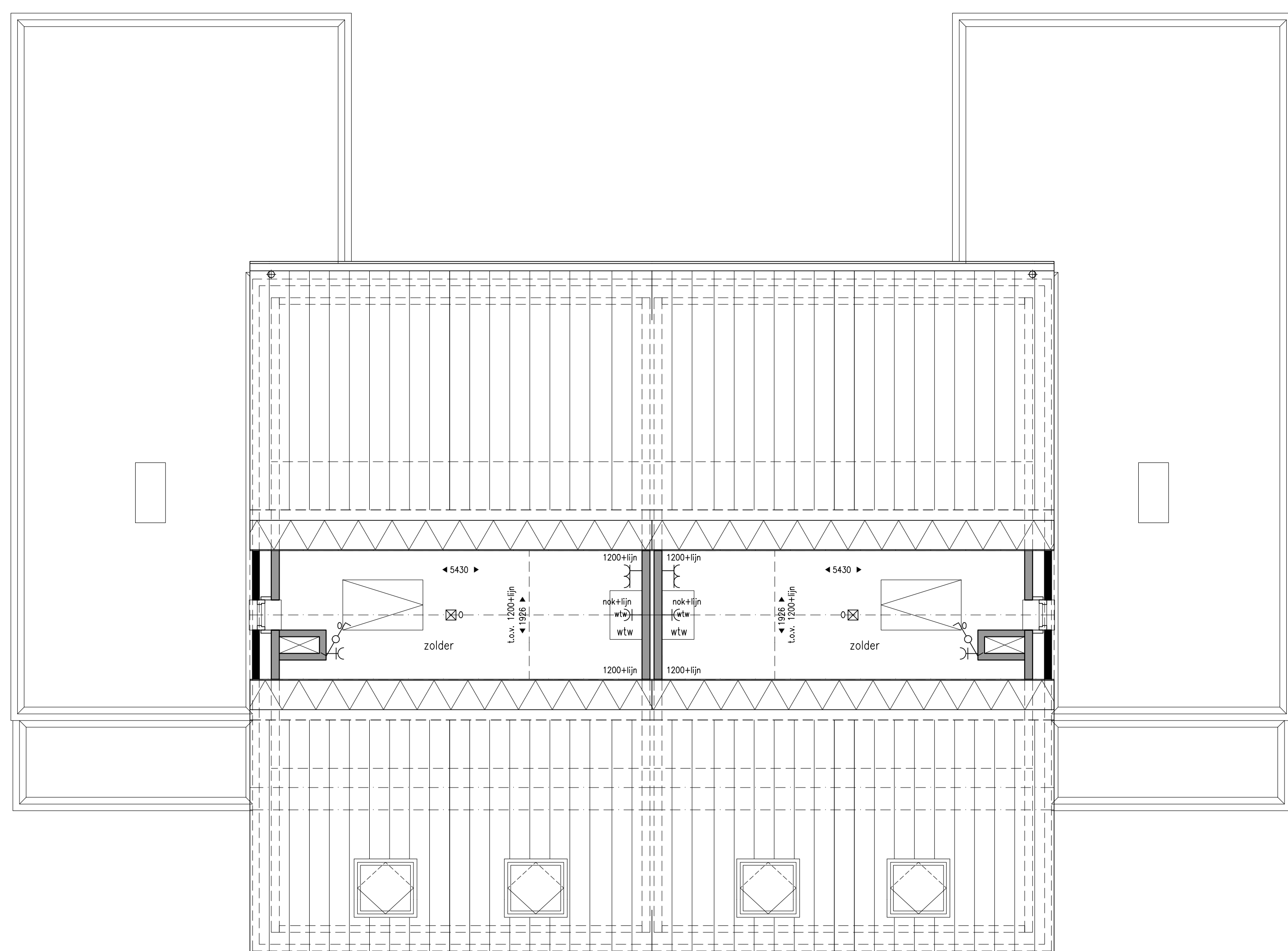
2e VERDIEPING 1:50
