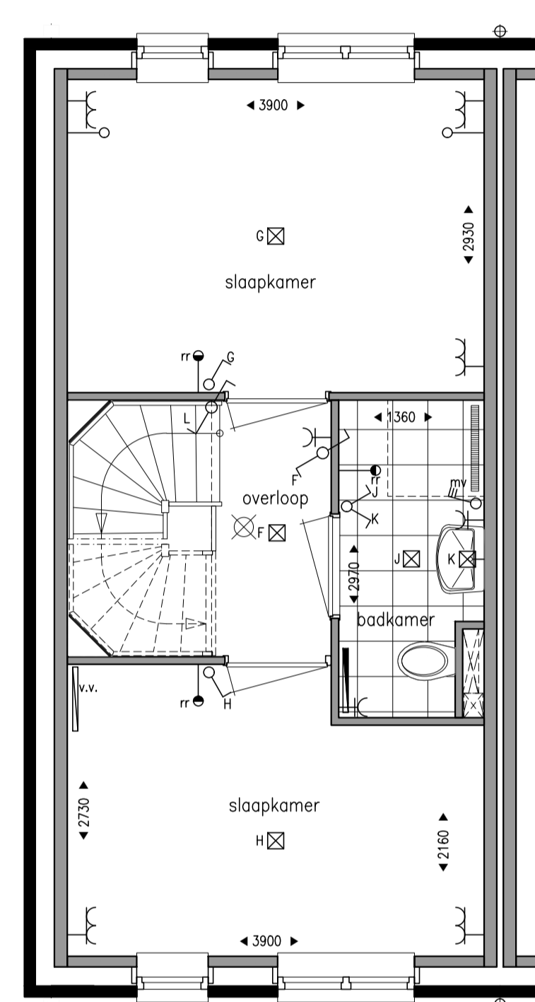
1e VERDIEPING 1:50
