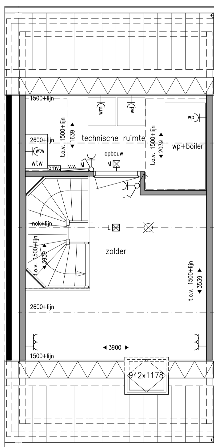
2e VERDIEPING 1:50
