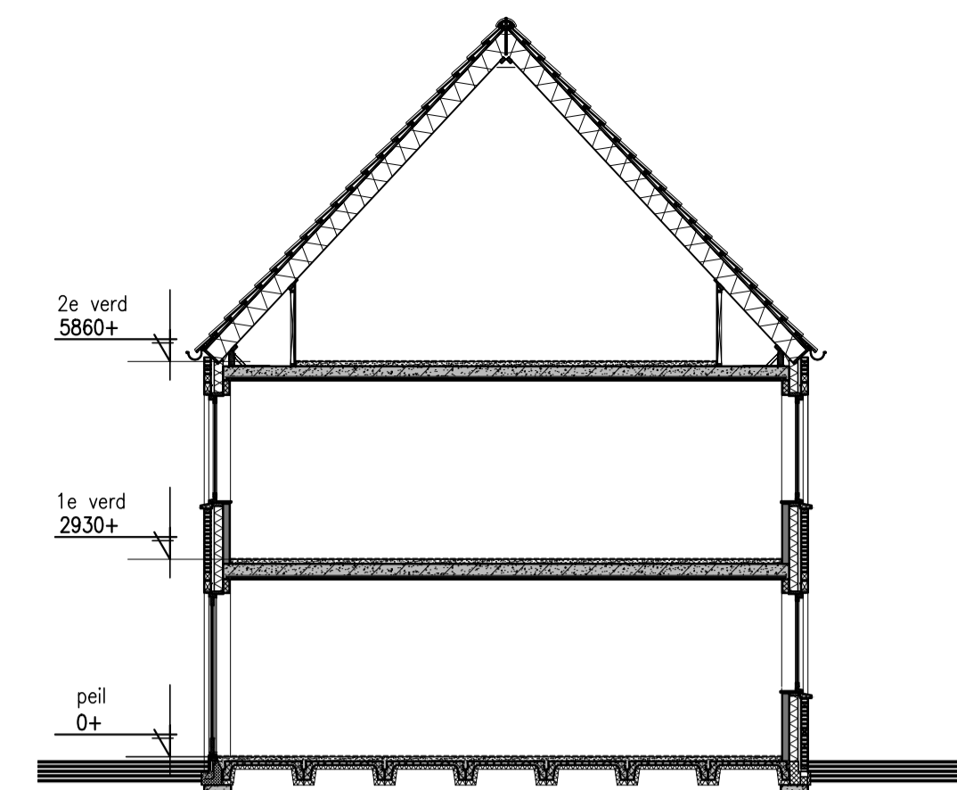
DOORSNEDE 1:100
