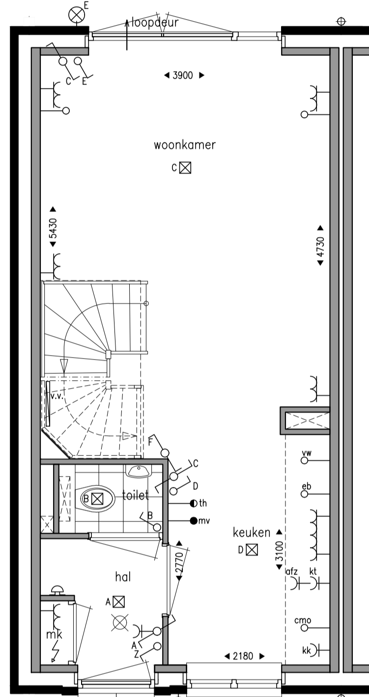
BEGANE GROND 1:50
