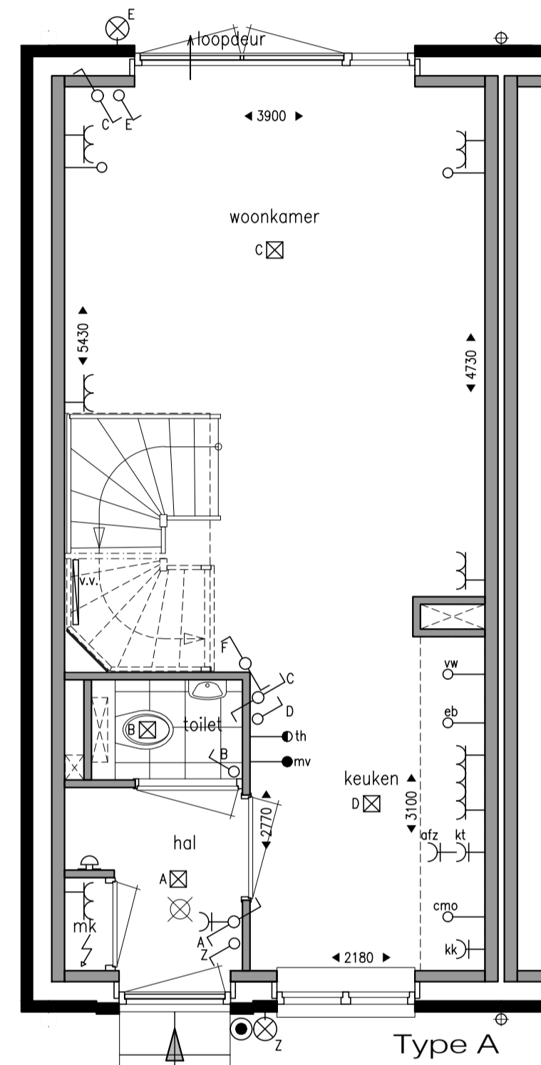
BEGANE GROND 1:50
