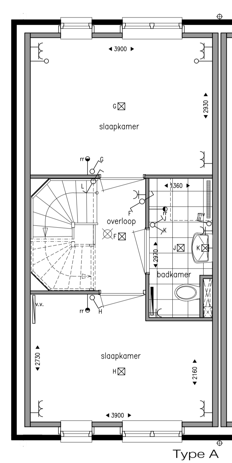
1e VERDIEPING 1:50
