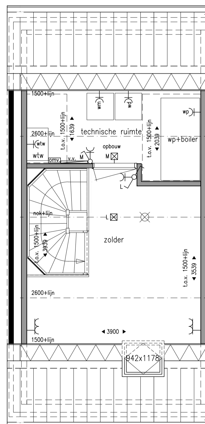
2e VERDIEPING 1:50
