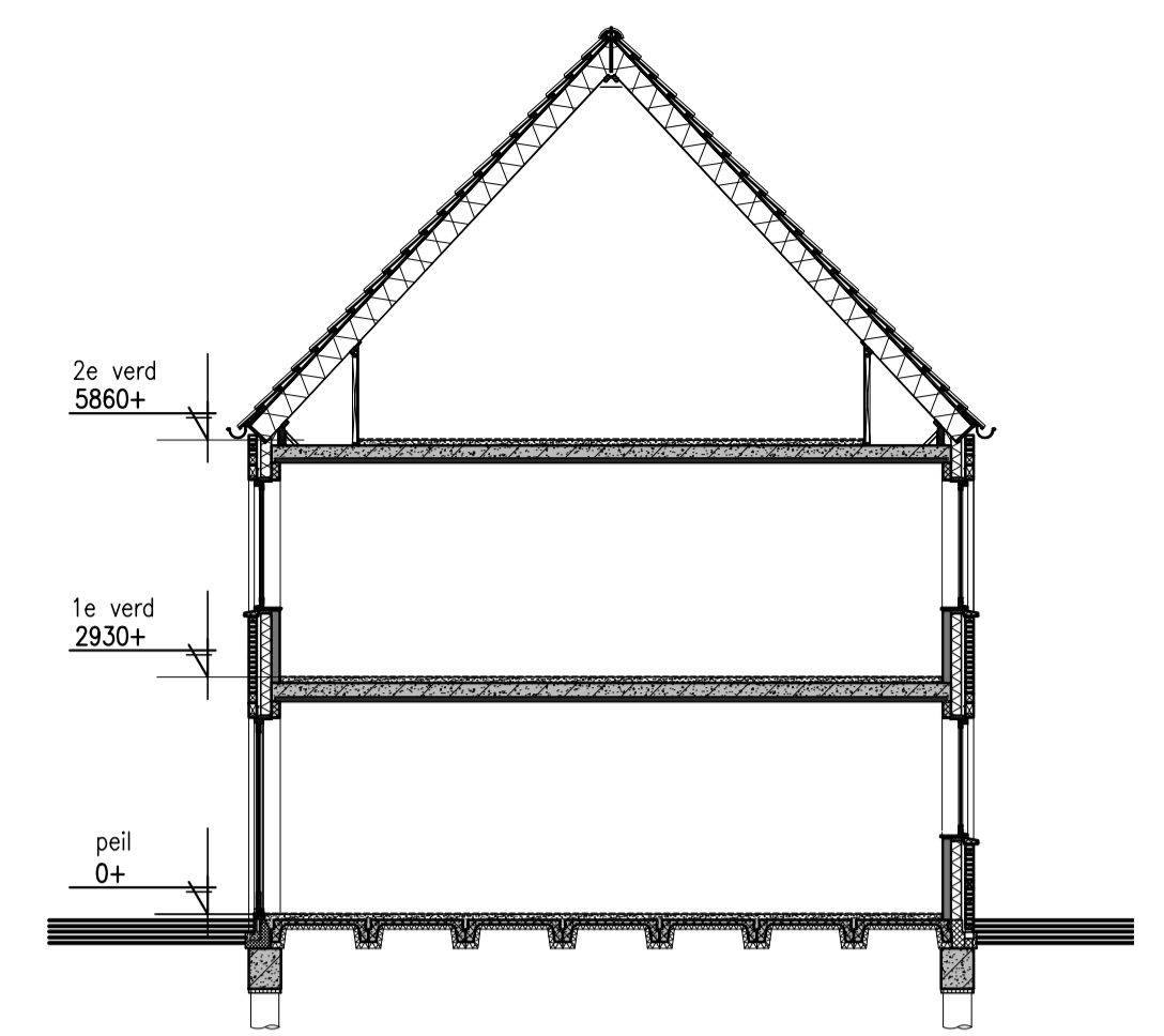
DOORSNEDE 1:100
