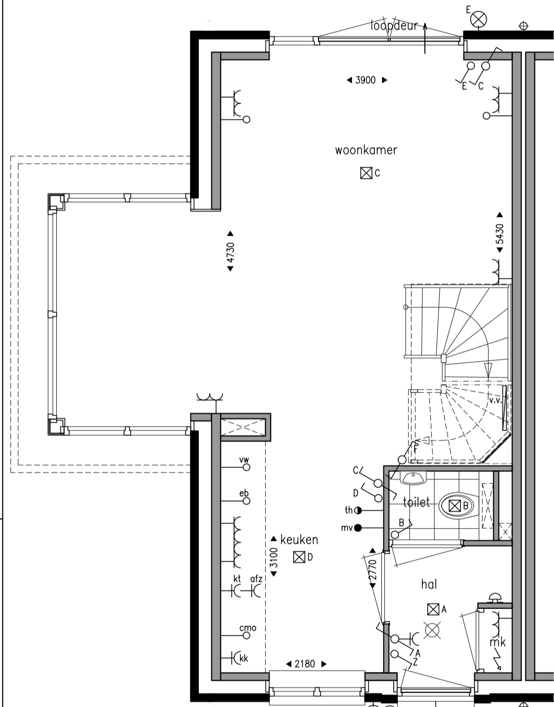
BEGANE GROND 1:50
