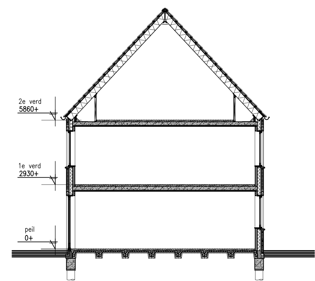
DOORSNEDE 1:100
