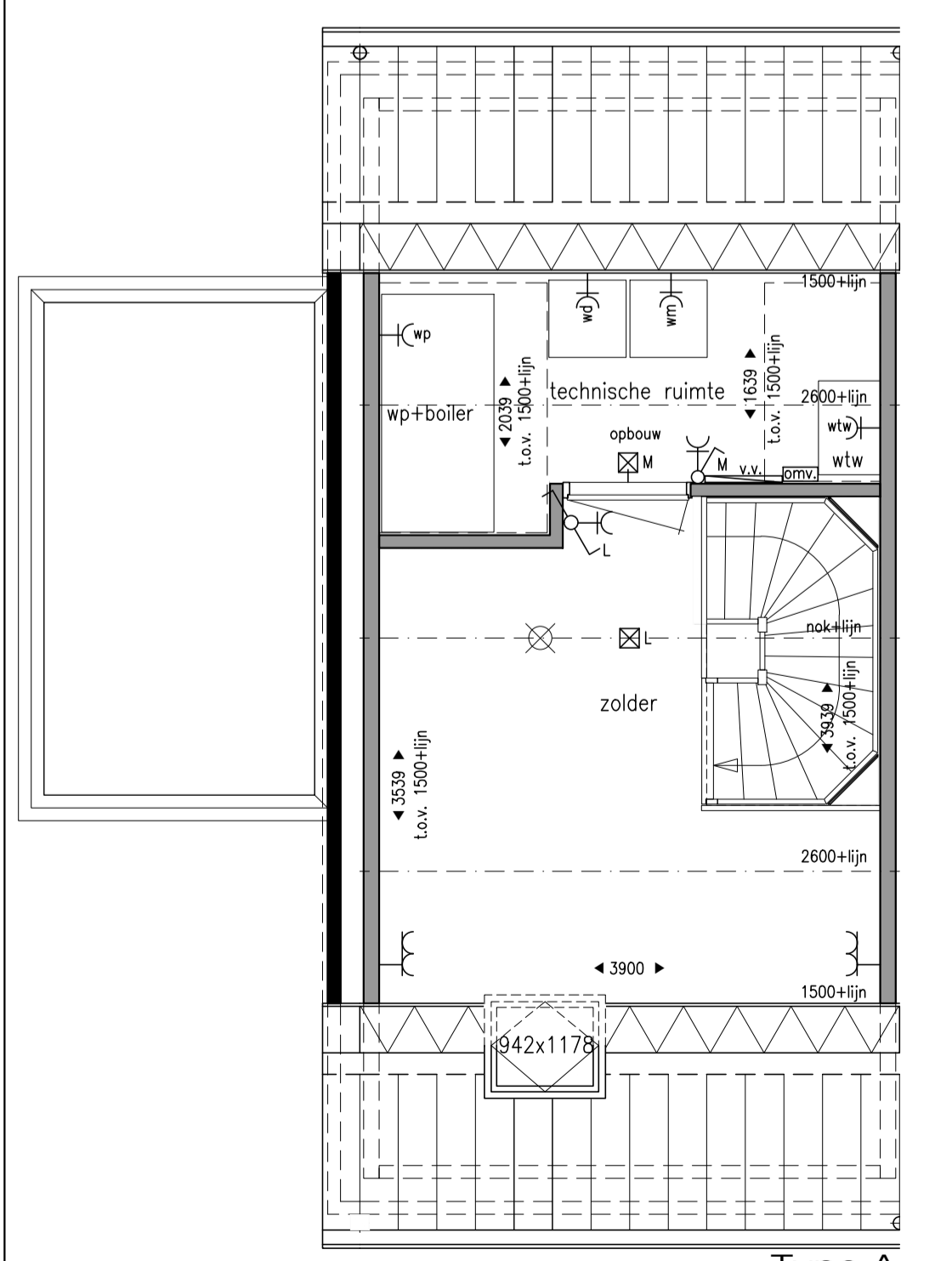
2e VERDIEPING 1:50
